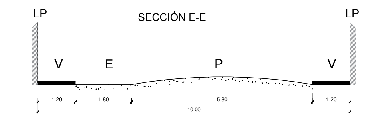
SECCIONES VIALES ESC. 1/50
